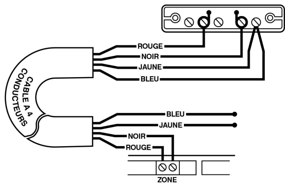
Figure 4 – Câblage des Contacts Magnétiques
